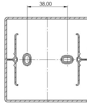
SCHNITT A-A
