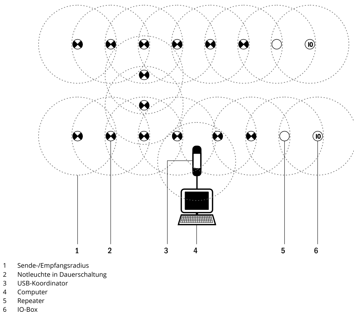
Abbildung 7: Aufbau eines WirelessProfessional-Systems
