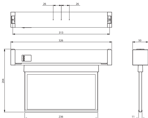
Dimensions KAMU
