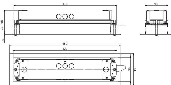
Dimensions KWIE recessed frame
