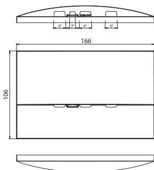
WEF Dimensions
