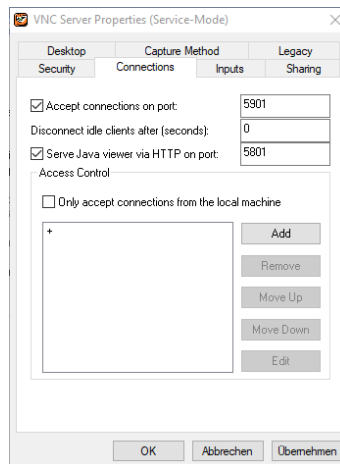
Abbildung 100: TigerVNC Server connections
