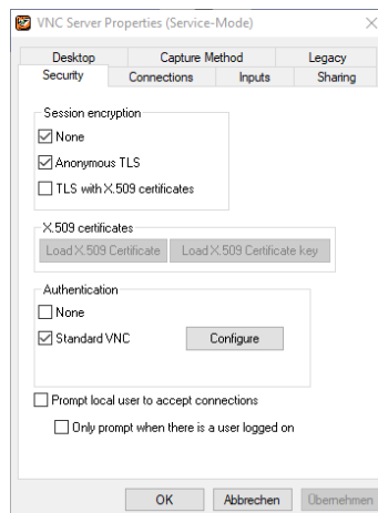
Abbildung 99: TigerVNC Server Einstellungen
