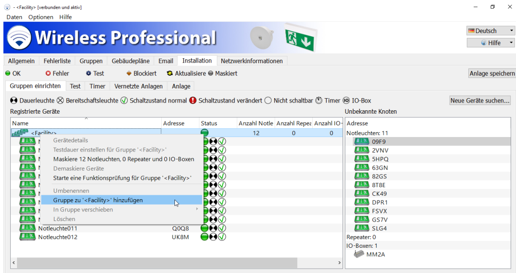
Abbildung 20: Erstellen einer Gruppe
