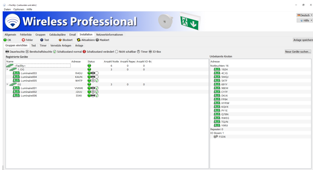
Abbildung 22: Geräte den Gruppen zuordnen
