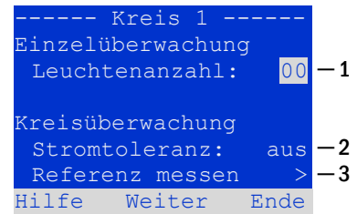
Abbildung 23: Stromkreisüberwachung einstellen
