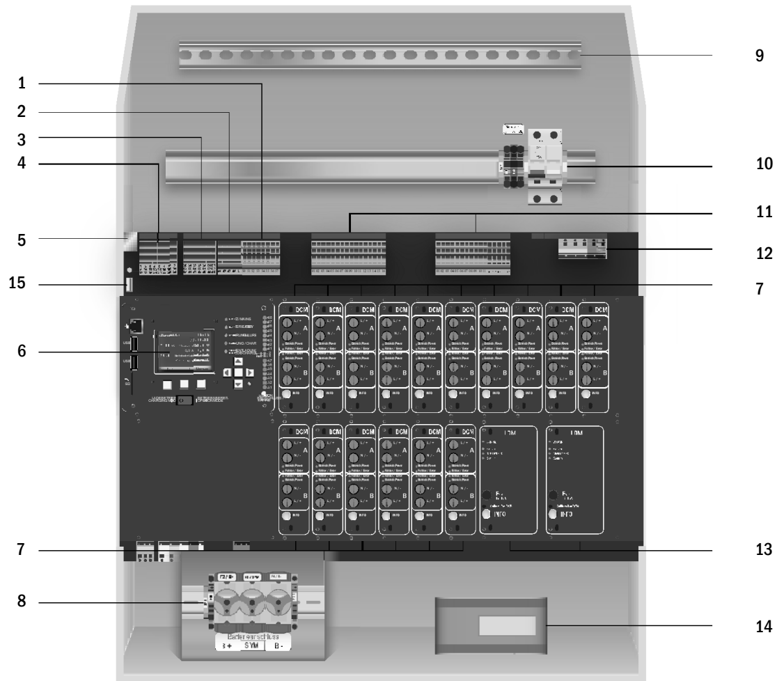
Abbildung 1: Innenansicht
