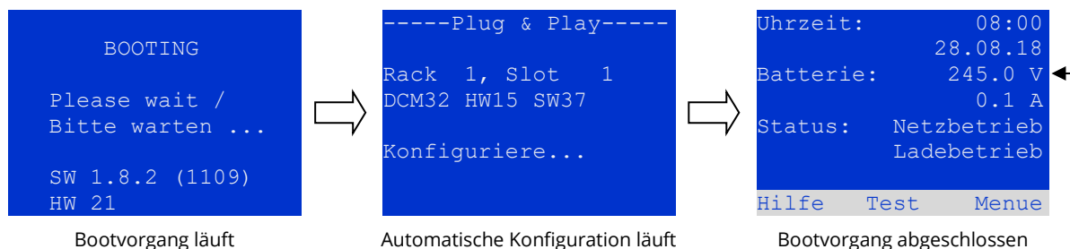
Abbildung 17: Bootvorgang (links, Mitte) und Statusanzeige (rechts).
