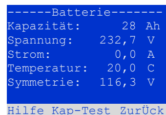
Abbildung 40: Batteriezustand
