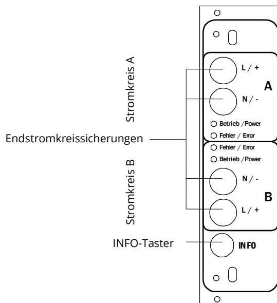
Abbildung 14: Stromkreismodul
