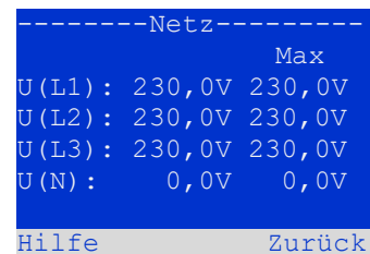
Abbildung 41: Zustand der Netzversorgung
