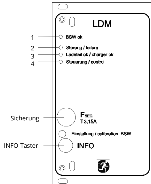
Abbildung 15: Lademodul LDM25
