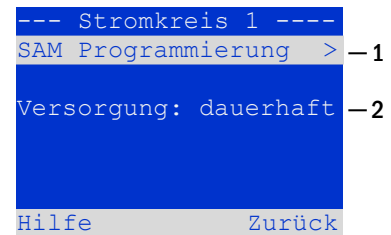
Abbildung 24: SAM-Programmierung
