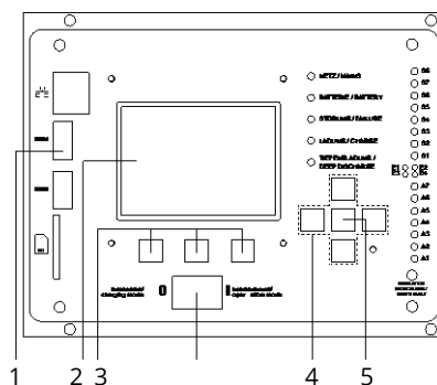
Abbildung 19: Bedienelemente
