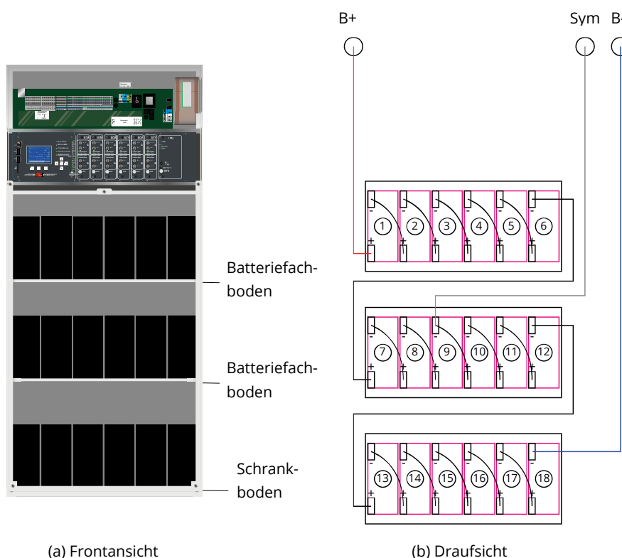
Abbildung 15: Aufstellung und Verschaltung der Batterieblöcke
