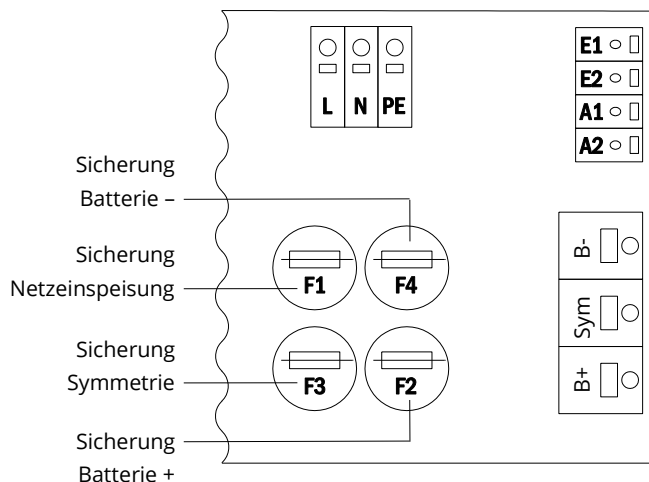
Abbildung 10: Sicherungen Netz- und Batterieeinspeisung
