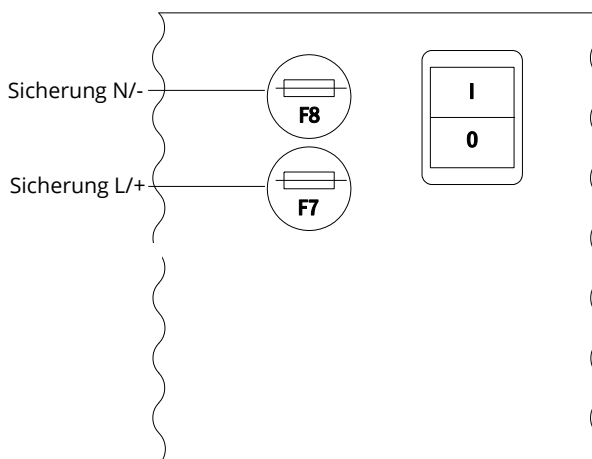
Abbildung 7: Sicherung Hilfsstromkreis
