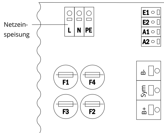
Abbildung 8: Netzeinspeisung
