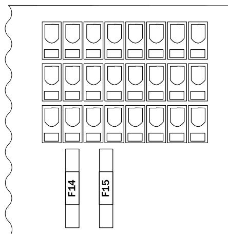
Abbildung 11: Sicherungen F14 + F15
