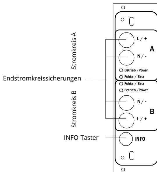
Abbildung 17: Stromkreismodul
