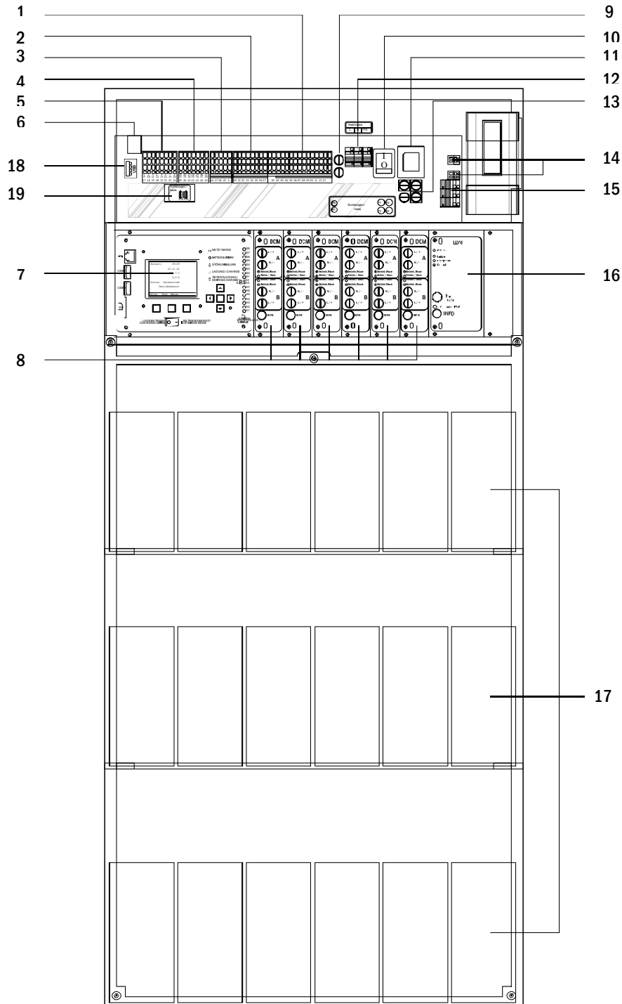
Abbildung 1: Innenansicht
