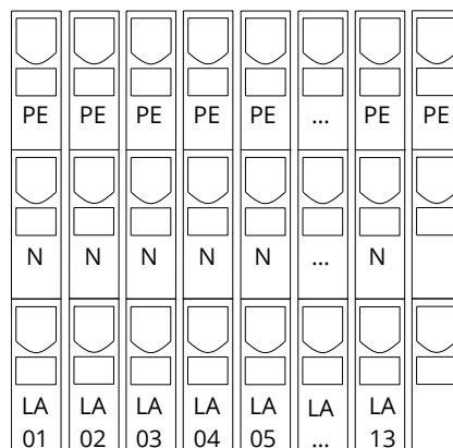
Abbildung 6: Stromkreise
