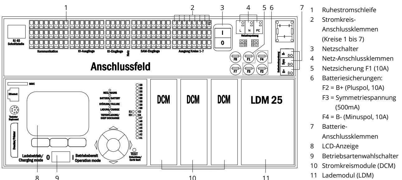
Abbildung 1: Ansicht der geöffneten microControl plus-Anlage
